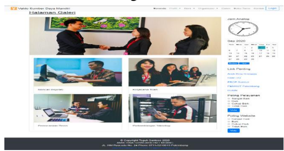
Gambar 4.12 Halaman Galeri
